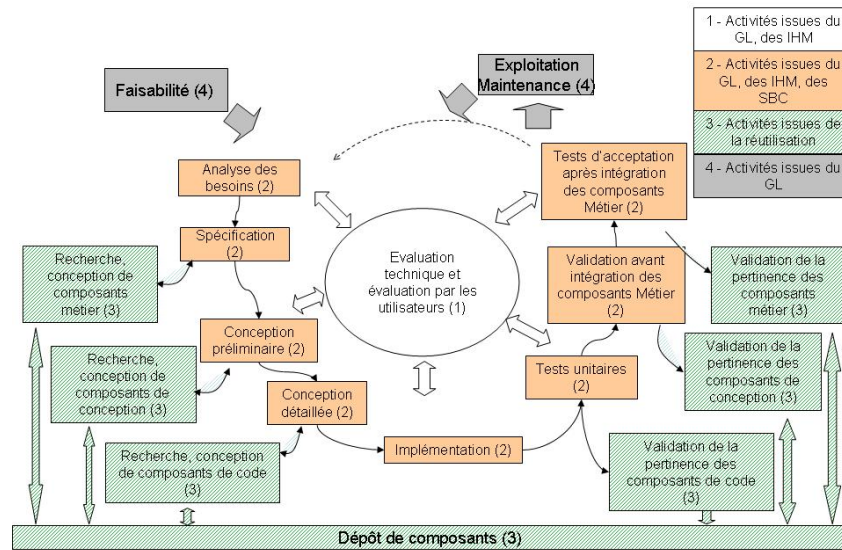
Figure 2. Le modèle d'ADESIAD, vue détaillée
