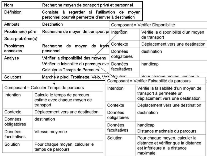
Figure 10. Composants, présentés par des patrons de composants, associés au sous-problème de recherche d'un moyen de transport privé et personnel, mis sous la forme de patron de problème
