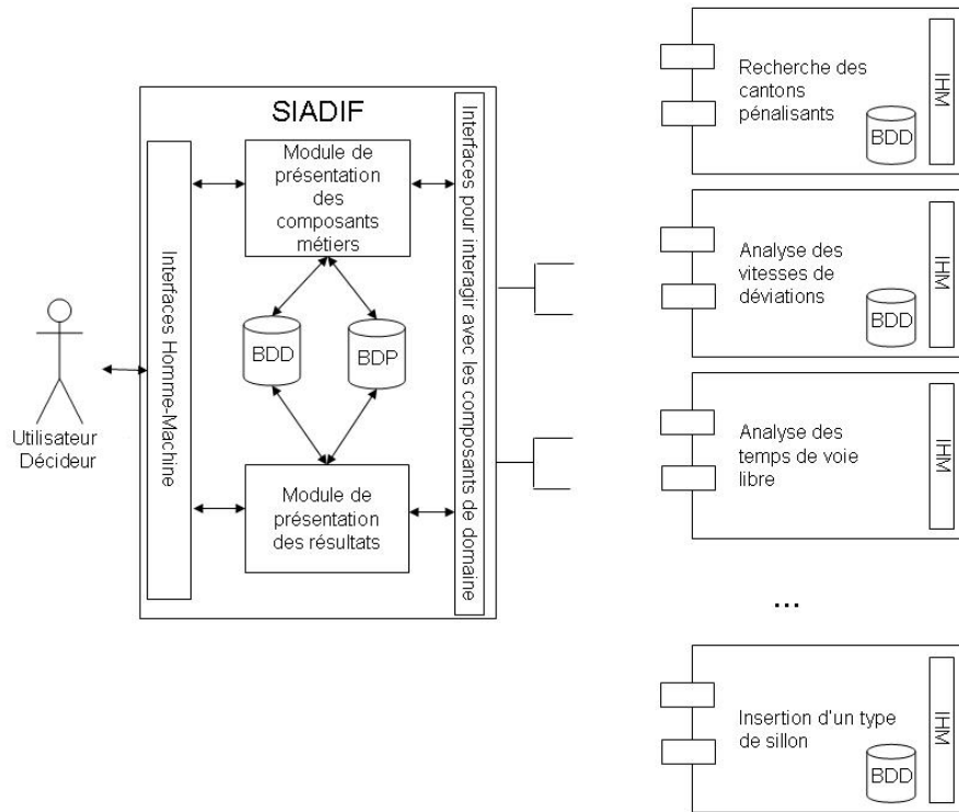
Figure 20. Description des modules du SIAD et positionnement des composants métiers
